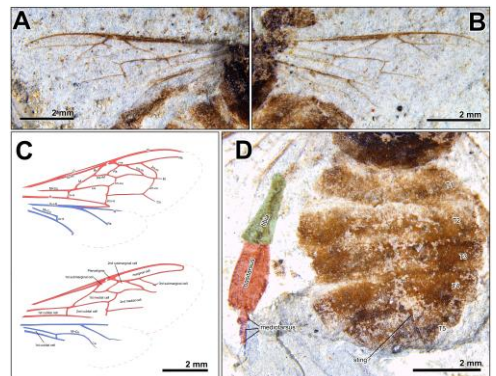
図2 タジマミツバチの化石（翅と後脚） と翅のスケッチ
