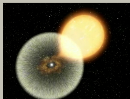
爆発する星“新星”の想像図 (イラスト提供： NASA JPL)
